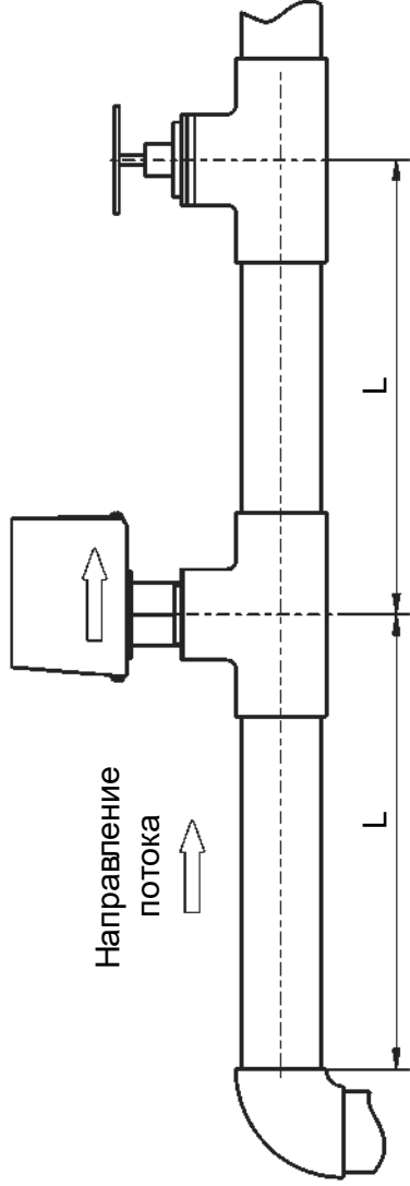
Расстояние "L" до ближайшего изгиба, вентилиа или любого фитинга должно быть не менее 5 диаметров трубы.
